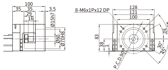
电机连接法兰 F1(台达\三菱400W)
