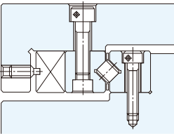
图3 间隙调节例
