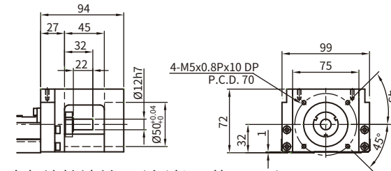
电机连接法兰 F1(台达\三菱750W)
