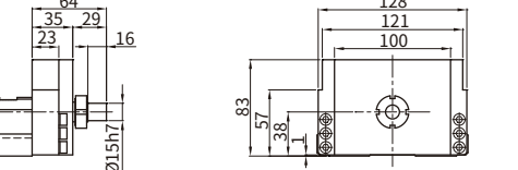
转接固定座 H0
