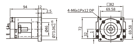
转接固定座 H0
