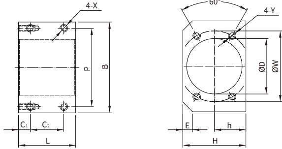
(2)BSG大导程螺母座
