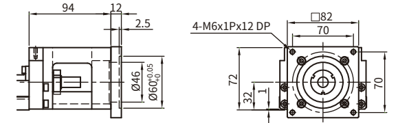
电机连接法兰 F4(86步进)
