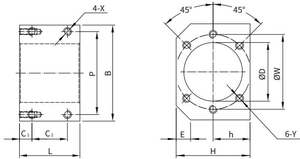
(1)DSGH螺母座
