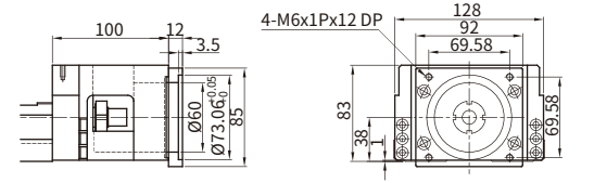
电机连接法兰 F4(松下750W)
