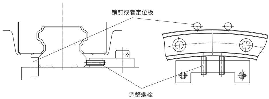
图4 押板固定
