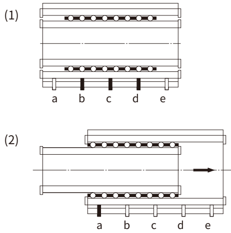
图2 调整螺栓的锁紧顺序
